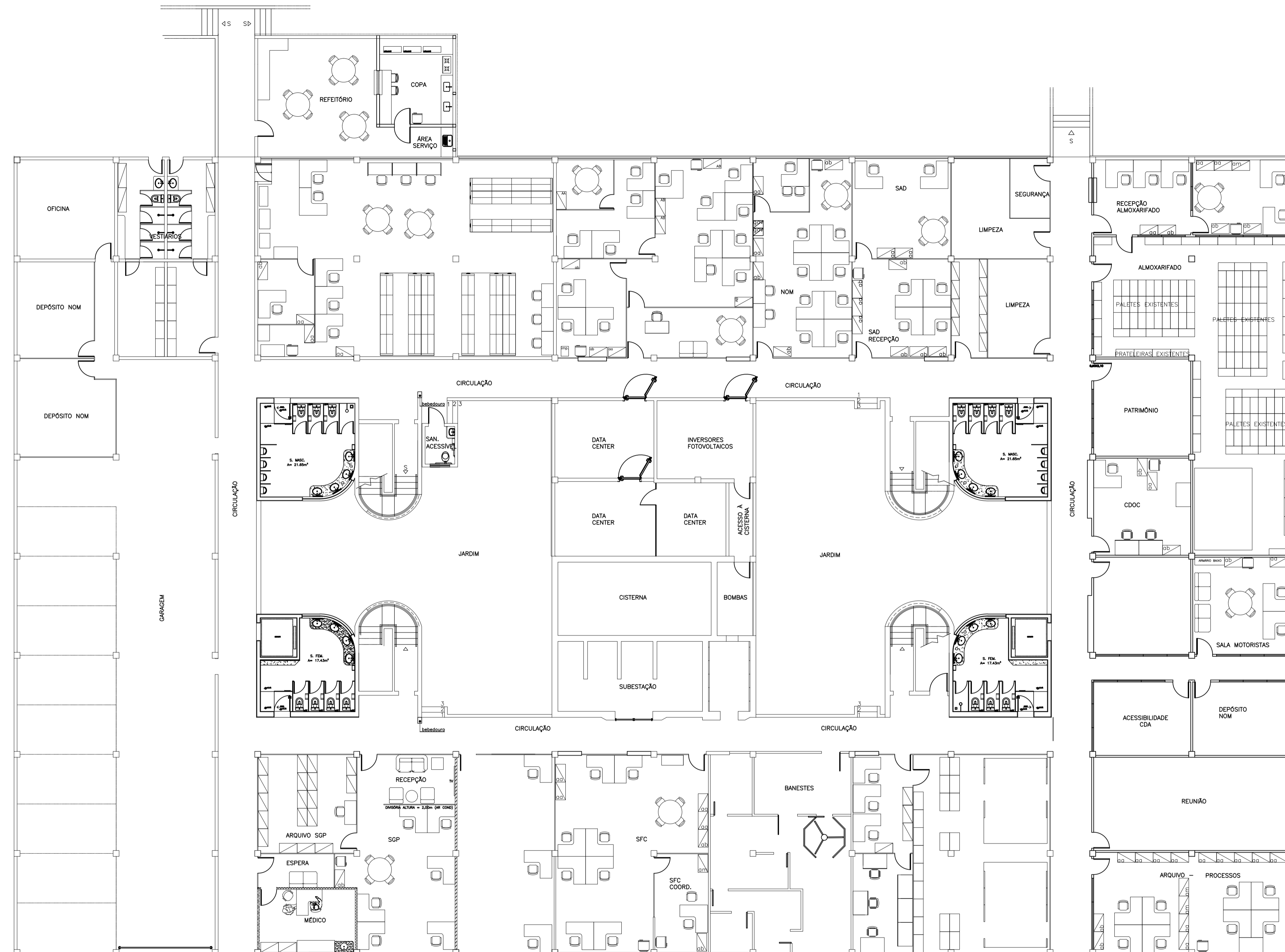
PLANTA BAIXA: PAVIMENTO TÉRREO ESCALA 1/125
